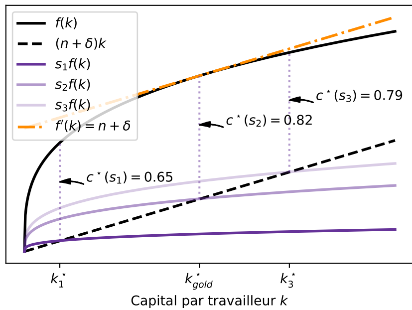
Figure 4.8: Condition d'optimalité
